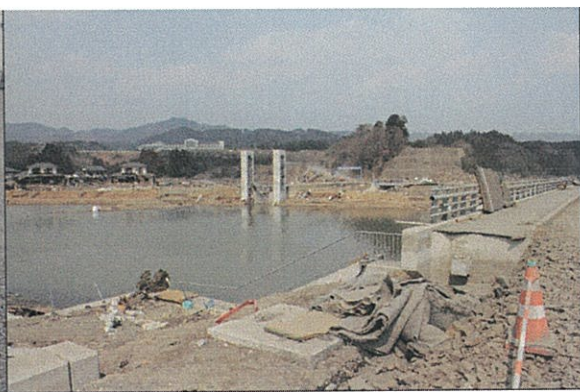
新追波橋より左岸の被災状況 大沢排水機場
